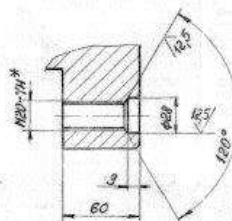
G-G (1:2)
